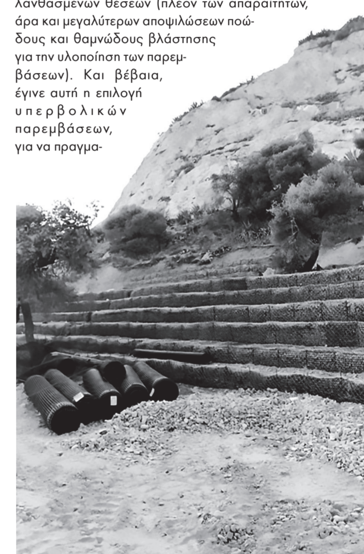
Φωτογραφία από τον Λυκαβηττό όπου βλέπουμε τον τρόπο συγκράτησης των πρανών με χρήση γεωπλεγμάτων και συρματοκιβωτίων. (01.08.2022)
